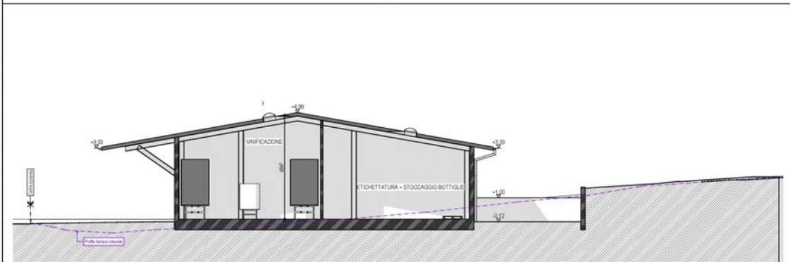
SEZIONE 2
